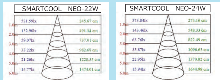
照度分布
